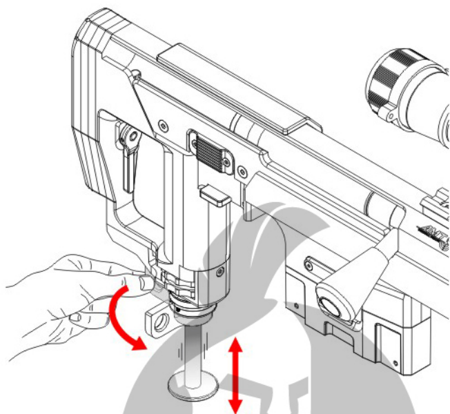
FAST EJECT
